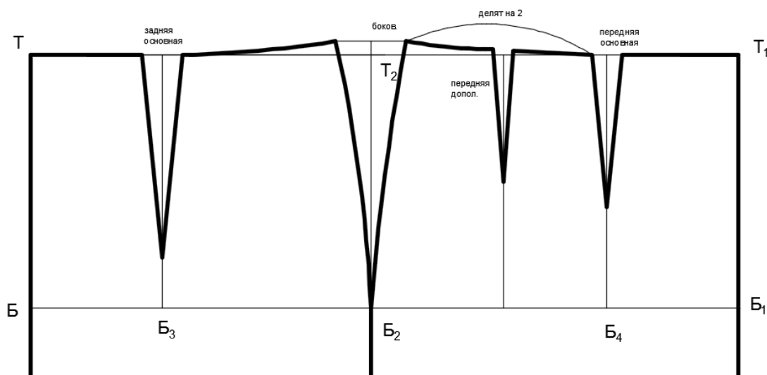
Рисунок 2 - Схема чертежа юбки с двумя талиевыми вытачками спереди (фигура с большим выступом живота)
