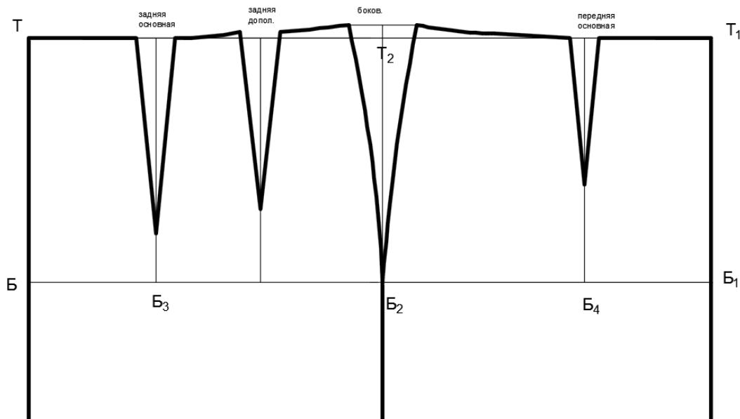
Рисунок 1 - Схема чертежа конструкции юбки с двумя вытачками сзади (фигура с выступающими ягодицами)
