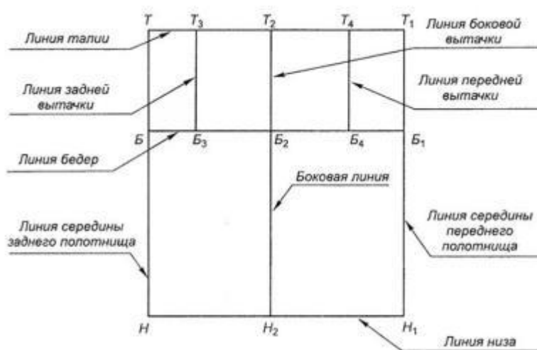
Рис. 2.2. Основа базисной сетки прямой юбки
