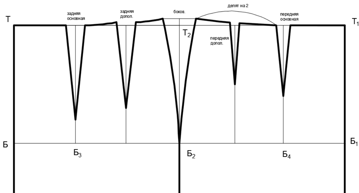
Рисунок 3 - Схема чертежа юбки с пятью талиевыми вытачками (фигура с узкой талией и широкими бедрами)
