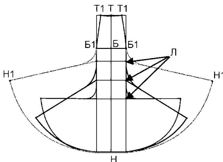
Рис. 2.. Схема чертежа конструкции клинневой юбки «годе»
