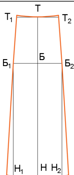
Рис. 1. Схема чертежа конструкции клинневой юбки
